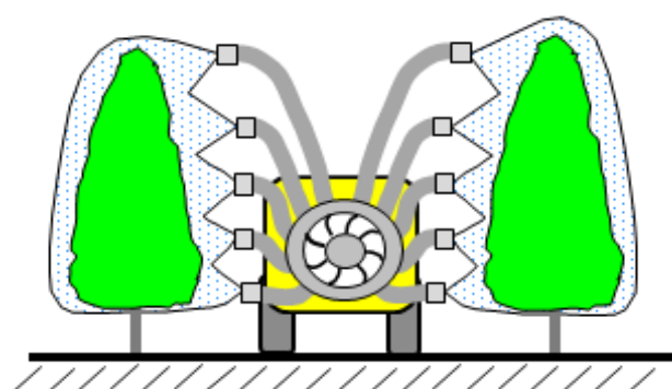
Opryskiwacz z wentylatorem promieniowym - kierowany strumień powietrza
