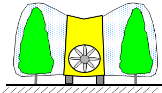
Opryskiwacz z wentylatorem osiowym z deflektorem
